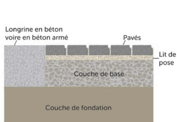
Figure 29 - Exemple de blocage des rives au moyen d'une longrine en béton.
