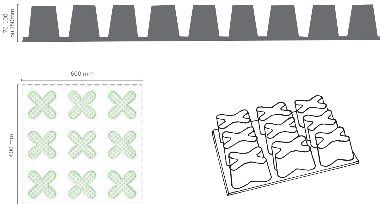
Figure 13 - Procédé Grasscrete, avec moules en plastique recyclé. Moules disponibles en épaisseur 76 mm, 100 mm et 150 mm.
