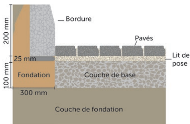
Figure 28 - Exemple de blocage des rives à l'aide de bordures et/ou de caniveaux.
