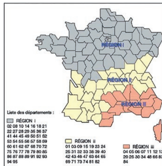
Figure 25 - La France en trois zones de pluviométries homogènes (extrait «Instruction technique», 1977)
