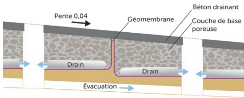
Figure 23 – Exemple de stockage sous chaussée et trottoirs à forte pente.
