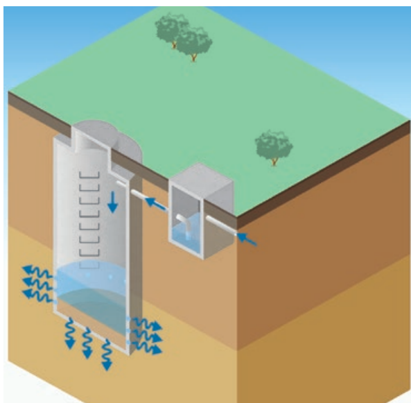
Figure 9 - Puits d'infiltration.
