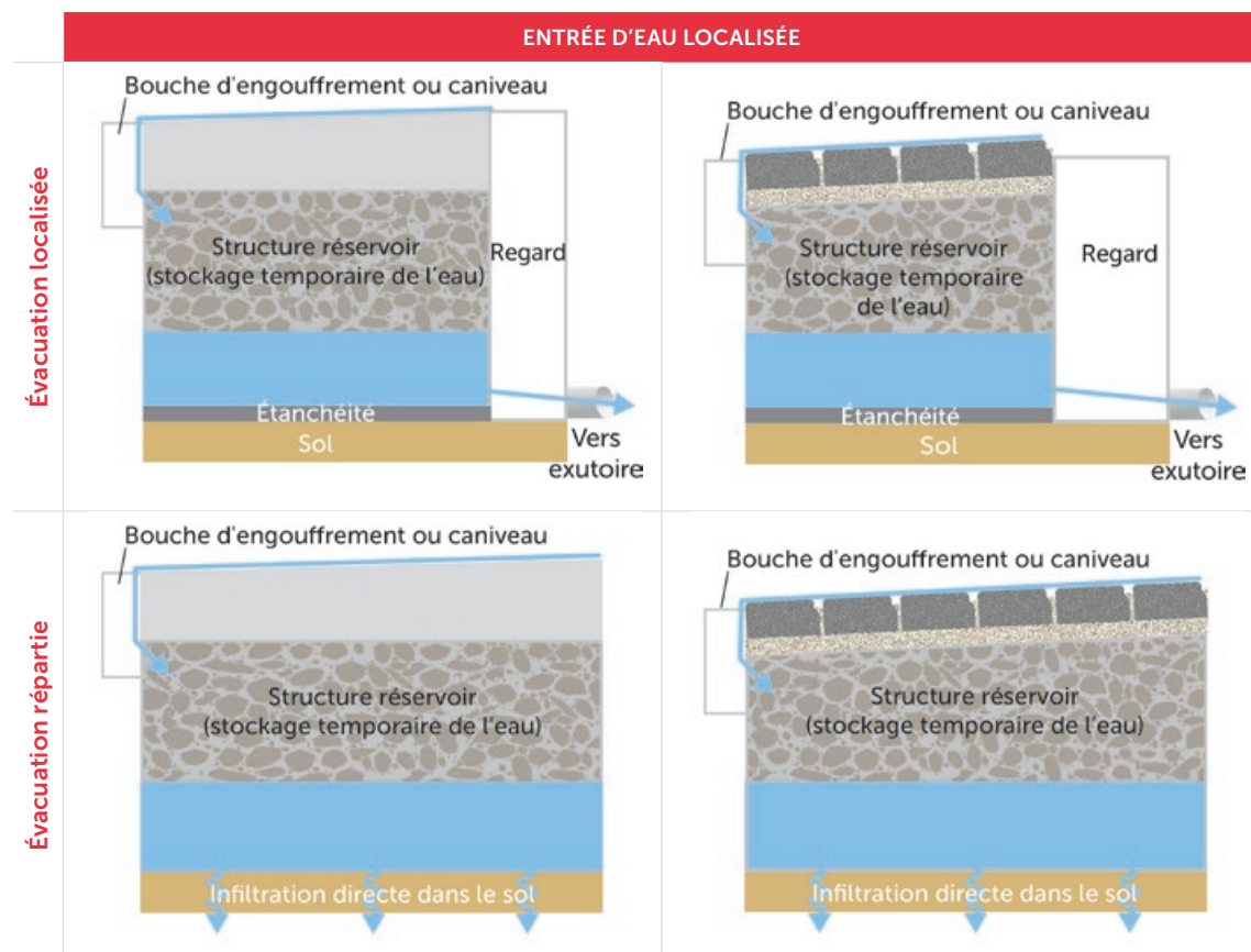
Figure 11 - Différents concepts de chaussées à structure réservoir avec entrée d'eau localisée.
